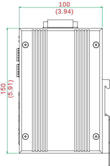
左侧视图
