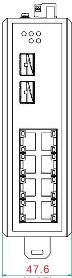
前视图
