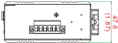
顶视图
