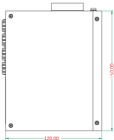
前视图
